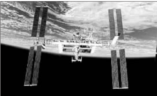
国际空间站
