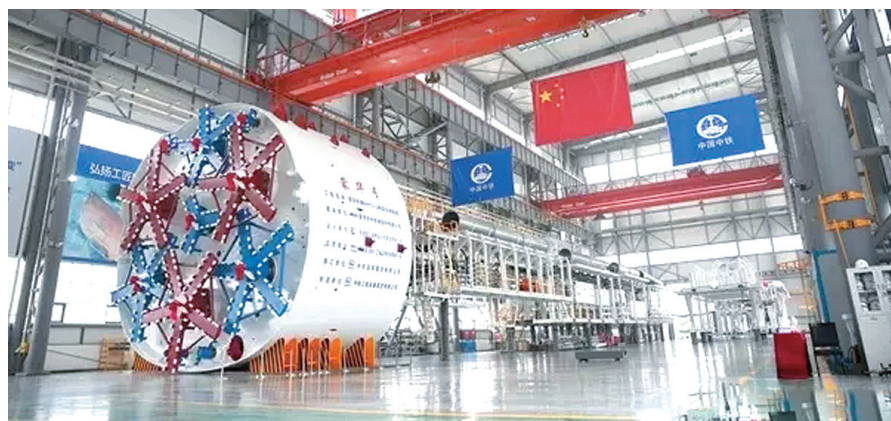
马蹄盾构
