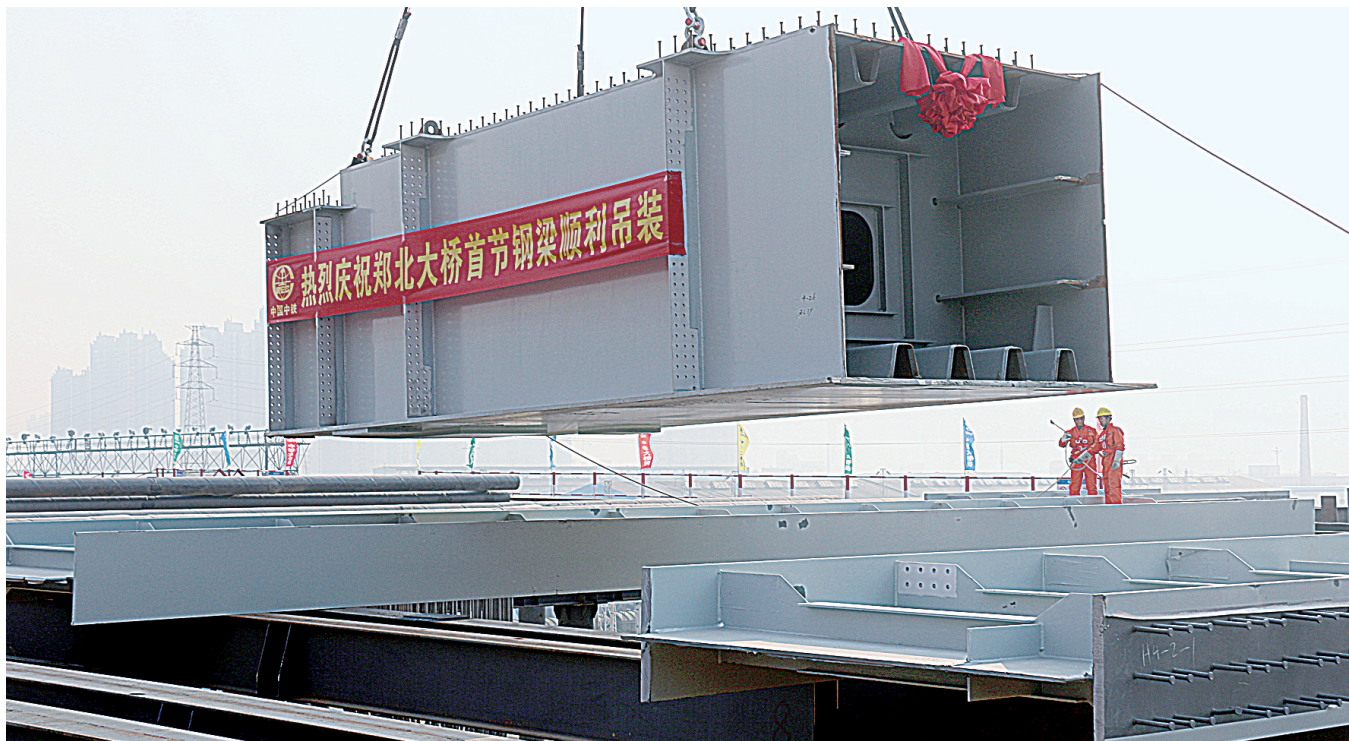
吊装现场
