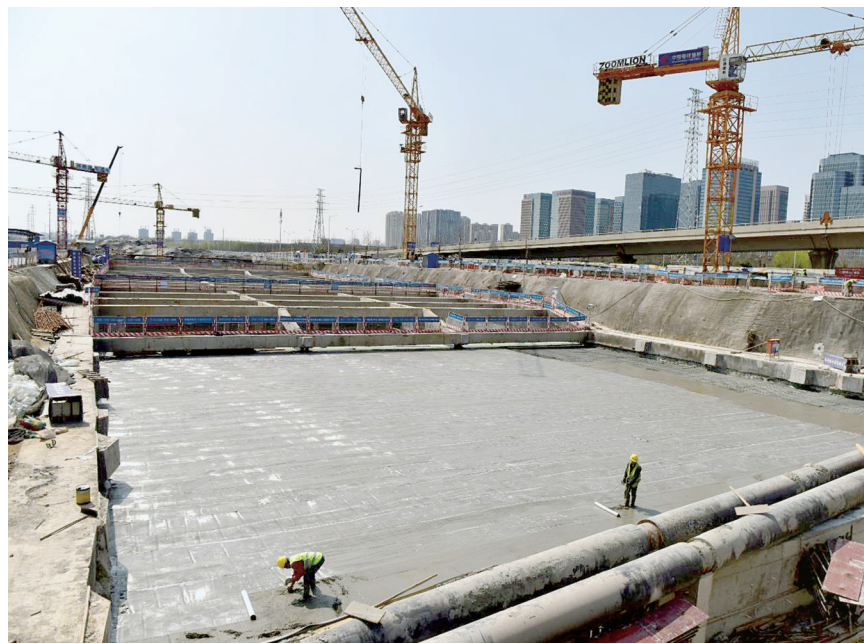
下穿隧道转入地面施工
