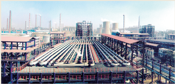
70万吨氧化铝项目管道化溶出系统。
