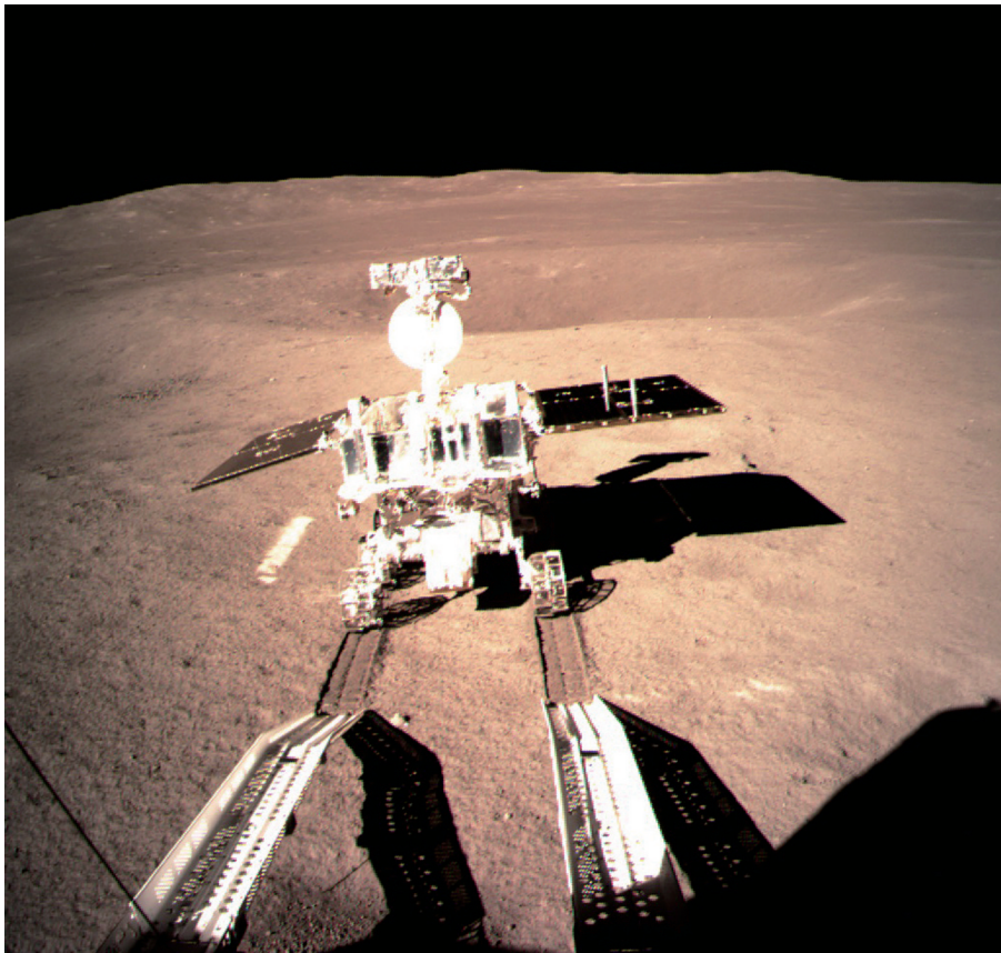
嫦娥四号着陆器监视相机C拍摄的玉兔二号巡视器走上月面影像图
