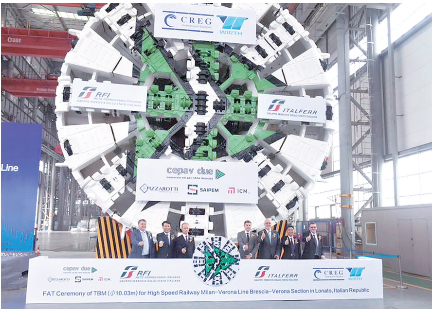
由中铁工程装备集团研制、出口意大利的大直径土压平衡盾构机22日在郑州成功下线。
