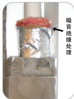
▲上海美巢装饰噪音绝缘处理工艺
