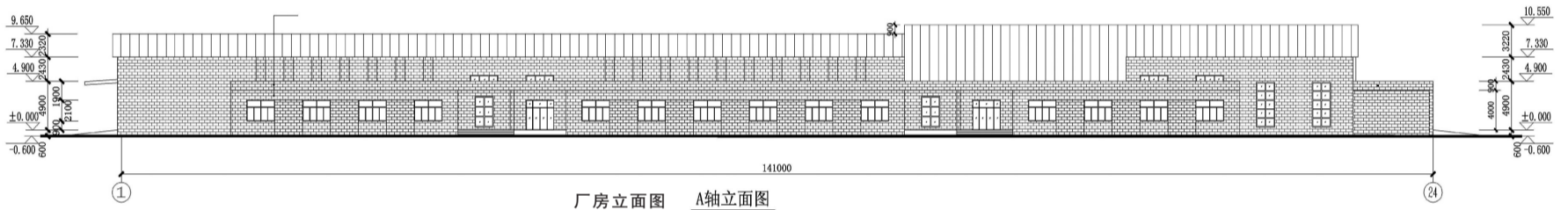
厂房立面图 A轴立面图
