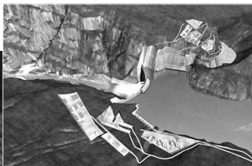
白鹤滩水电站示意图
