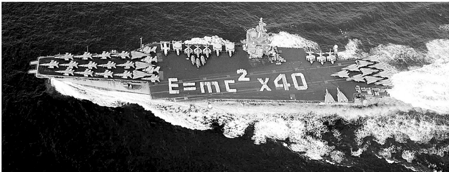
这张照片摄于2001年11月5日,水兵们在飞行甲板上摆出爱因斯坦著名的公式“ E = MC^2 \times 40 ”的字样,来纪念美国海军使用核动力水面舰船40周年。当时企业号完成“持久自由”行动,正在返回母港。
