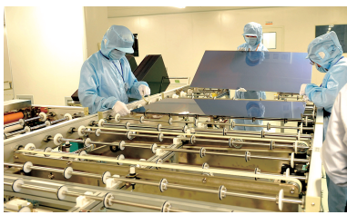
河南保绿能源非晶硅太阳能生产线
