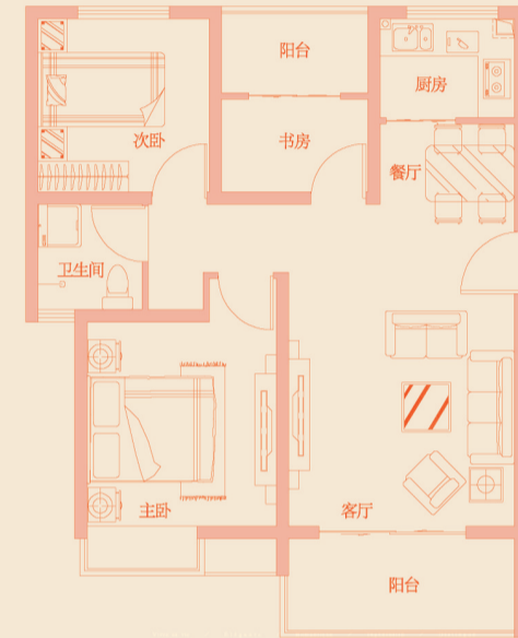
A-1 两室两厅一卫 户型 建筑面积约86.67m 2
