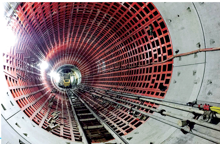
←2号线紫荆山站至东大街站盾构区间左线隧道顺利贯通。 郑州晚报记者 詹莉莉 图
