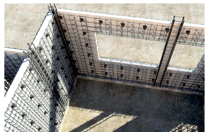
保温与结构一体化模板
