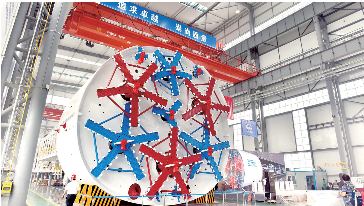
世界首台马蹄形盾构机在经开区成功下线 薛宁 图
