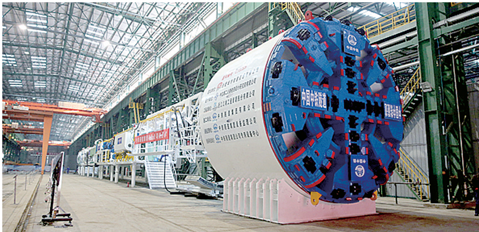
国内首台使用国产主轴承再制造盾构机顺利下线
