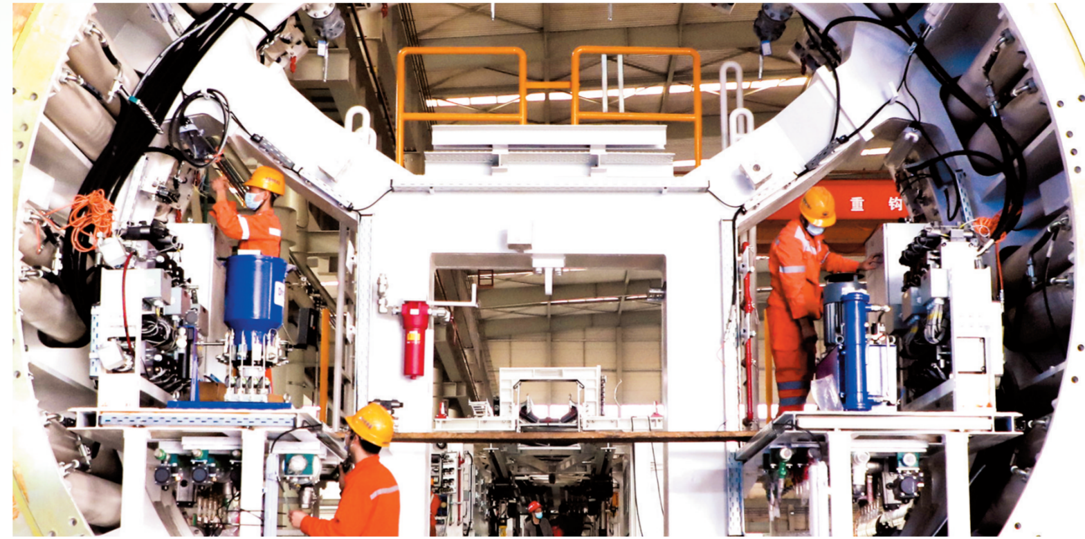
中铁装备工人组装盾构机
