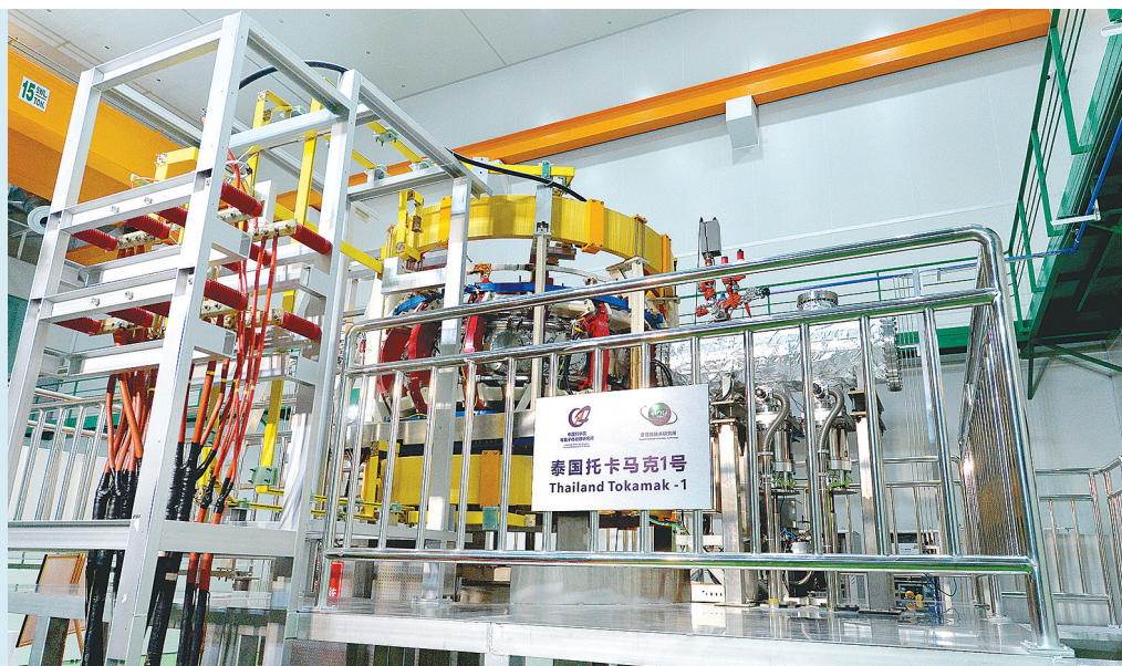
7月25日在泰国那空那育府拍摄的托卡马克实验装置 新华社发
