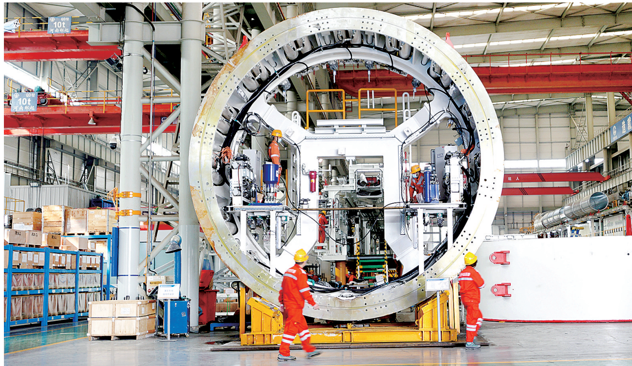
中铁装备工厂的盾构机制造现场
