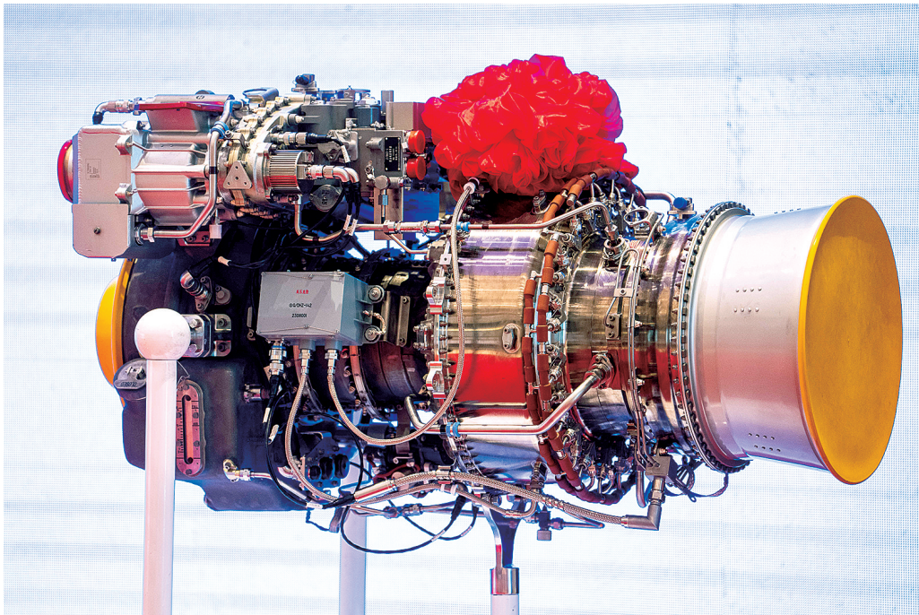
在AES100发动机研制工作总结会上拍摄的AES100发动机 新华社发
